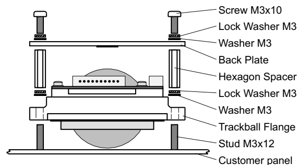
Fig. 1 : assembly procedure
