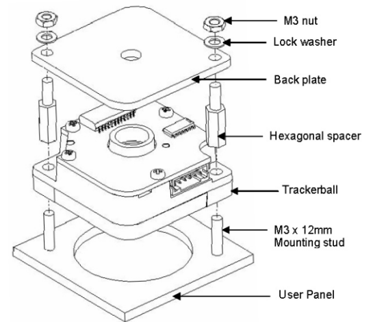
Fig. 1 : assembly procedure
